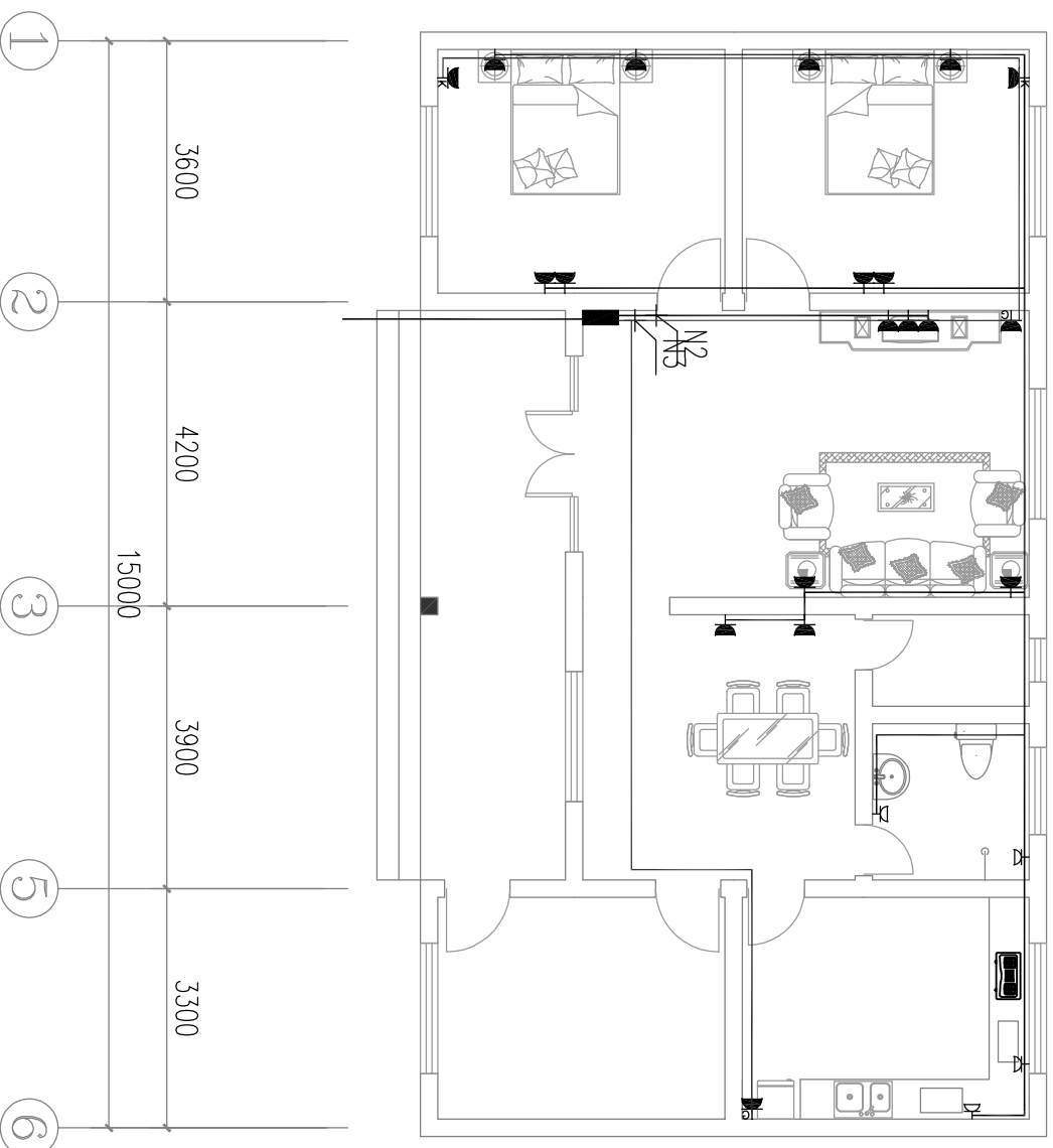
一层插座平面图 1:100
