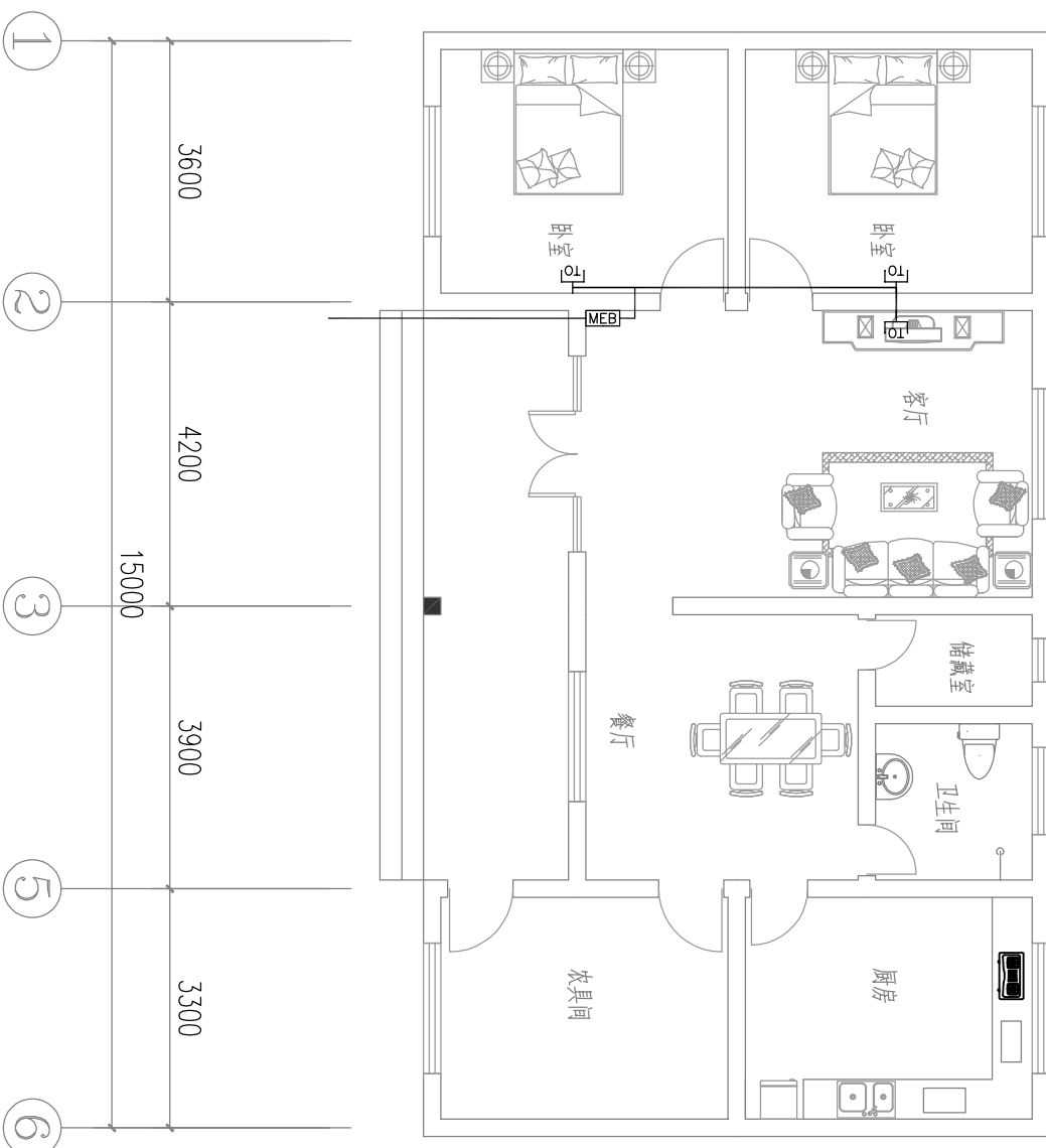
一层弱电平面图 1:100
