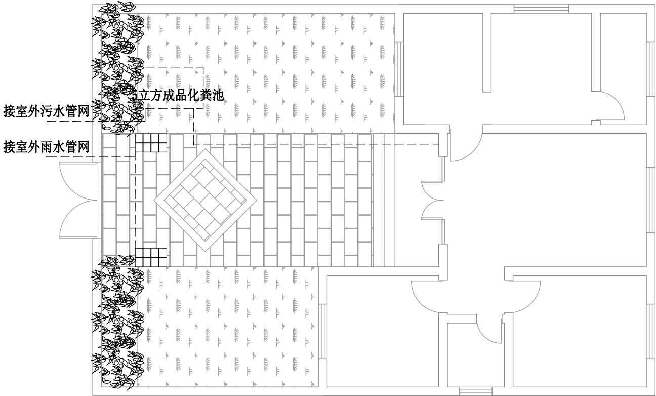
院落雨污水平面图 1:100
