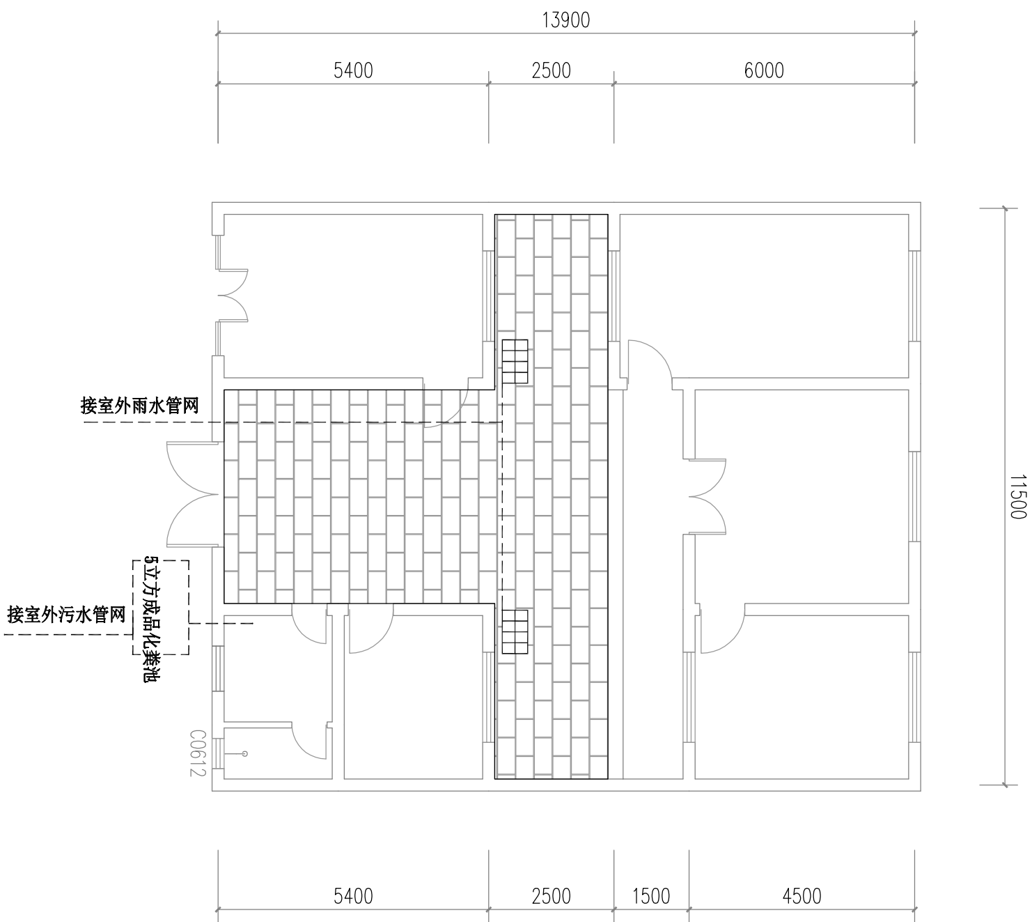
院落平面图 1:100
