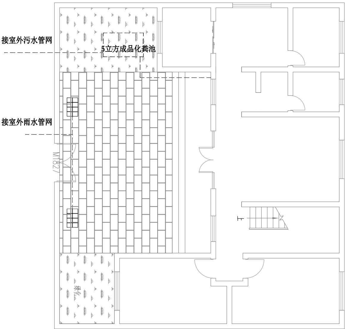
院落雨污水平面图 1:100
