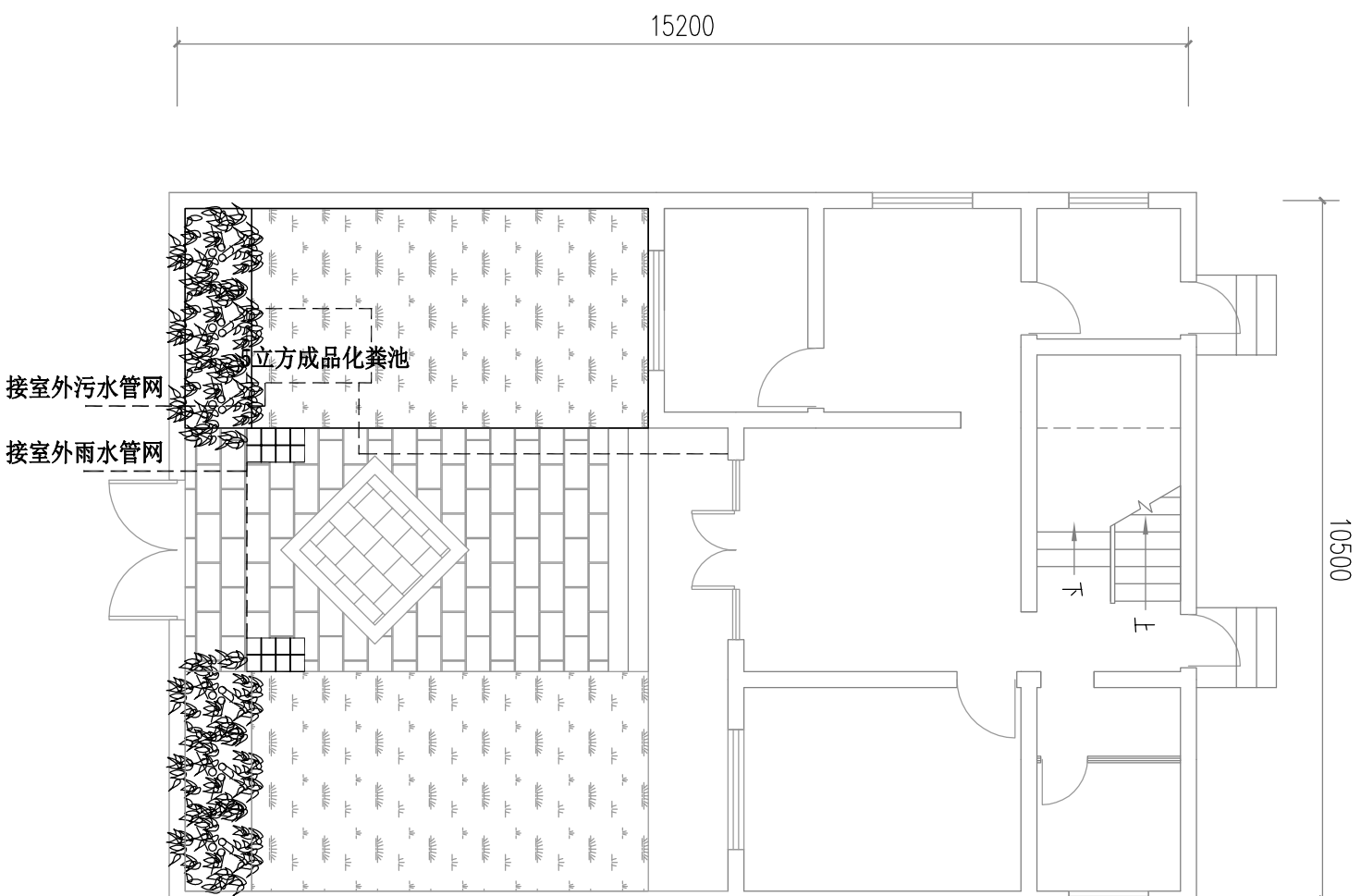
院落雨污水平面图 1:100
