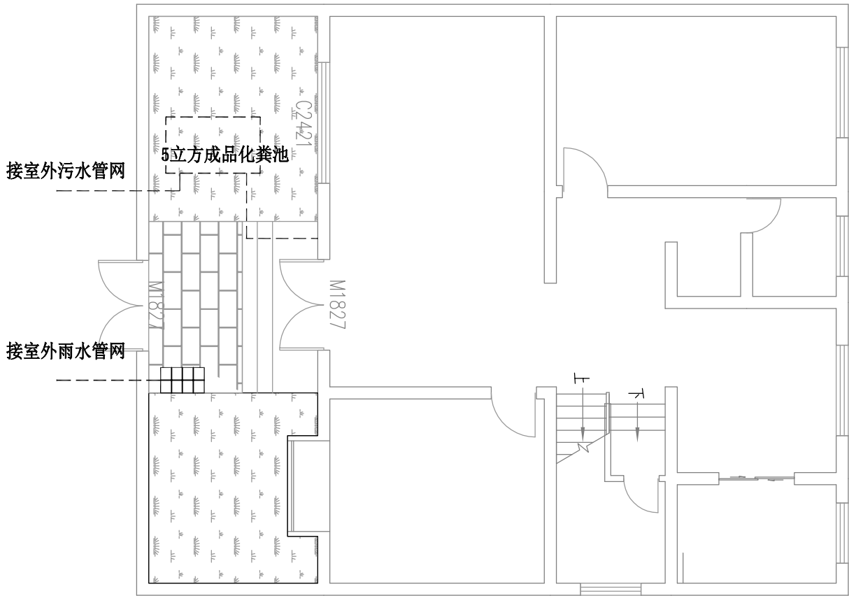
院落雨污水水平面图 1:100
